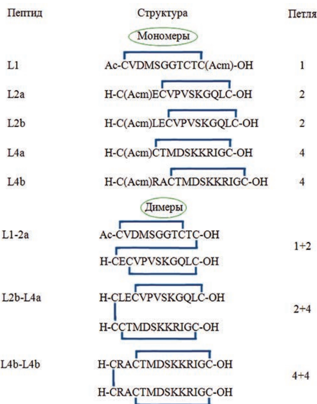
Рис. 5. Мономерные и димерные пептидные миметики 1, 2 и 4-й петель BDNF
