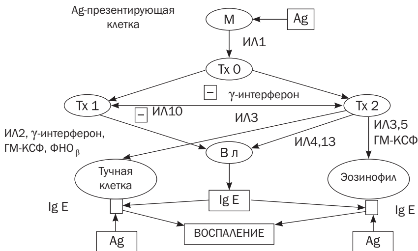
Рис. 6.1.1. Принципиальная схема воспалительной реакции тип 1
