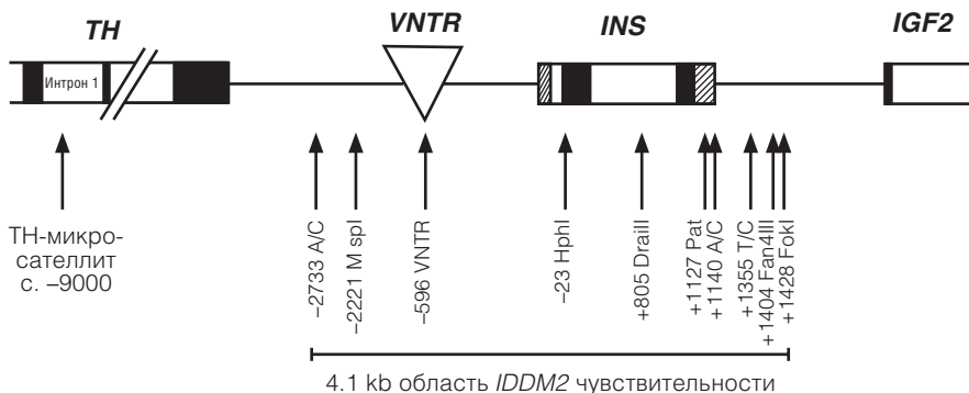
Рис. 6.3.7. Фрагмент хромосомы 11, содержащий ген инсулина
