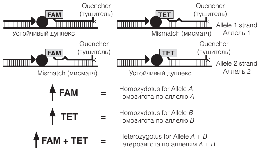
Рис. 4.5. Определение аллельного полиморфизма с помощью 5'-нуклеозного (TaqMan) анализа (пояснения в тексте)
