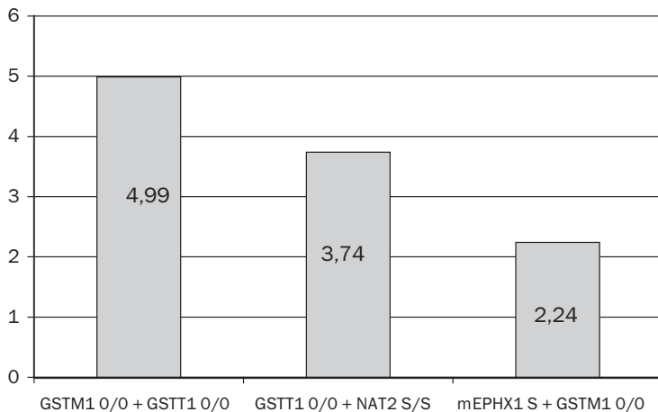
Рис. 6.6.5. Риск развития эндометриоза при сочетании двух функционально неблагоприятных генотипов
