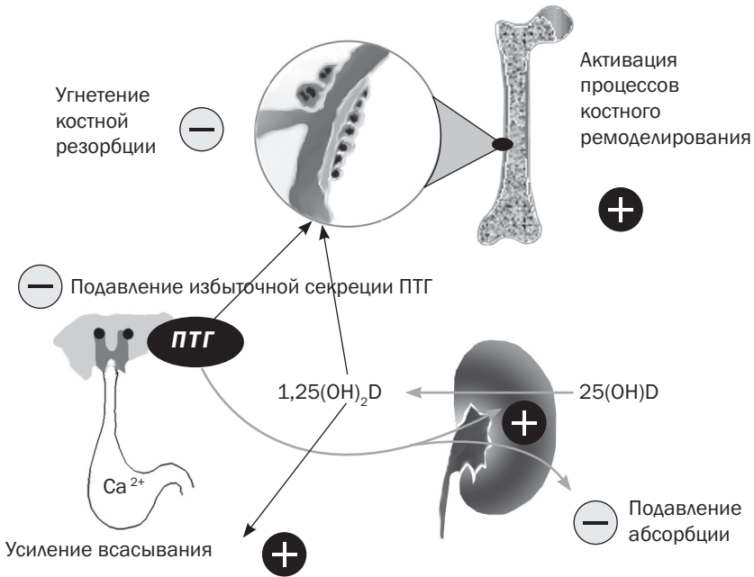
Рис. 6.2.3. Функциональная активность кальцитриола ПТГ — паратиреоидный гормон
