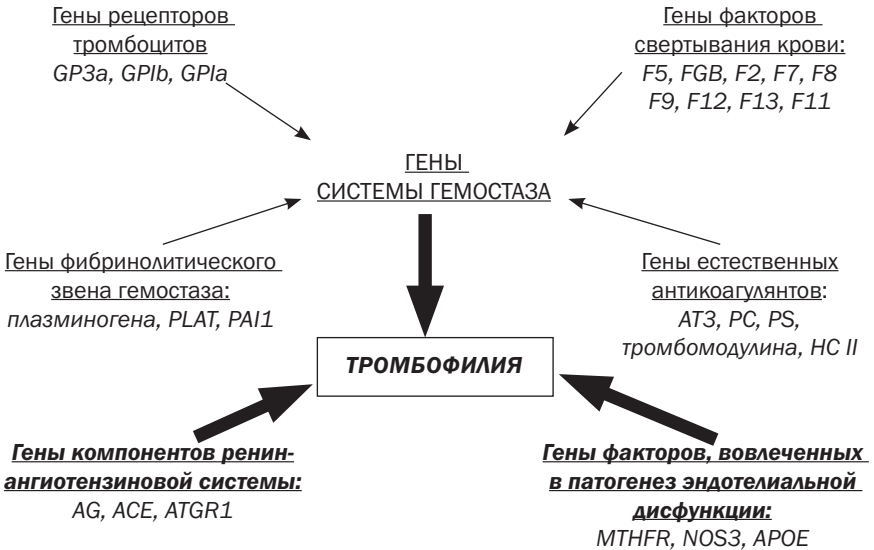
Рис. 6.6.27. Генная сеть тромбозии
