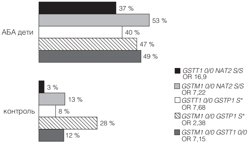
Рис. 6.1.6. Соотношения частот сочетанных генотипов по генам системы детоксикации у детей с атопической БА и у здоровых детей группы контроля
