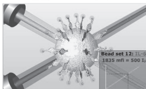
Рис. 4.20. Принцип детекции мутаций на микросферах ( www.perkinelmer.com ) (пояснения в тексте)
