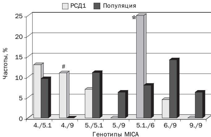
Рис. 6.3.6. Частоты генотипов MICA в группе риска (РСД1) и в контрольной группе. Примечание: * — достоверные отличия при p < 0,05 ; # — достоверные отличия при p < 0,01
