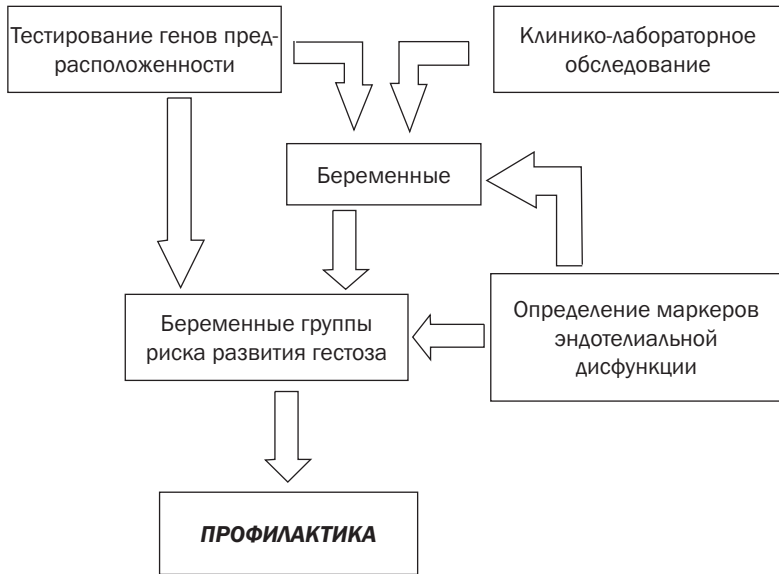
Рис. 6.6.25. Алгоритм профилактики гестоза [221]
