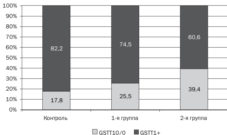
Рис. 6.6.8. Распределение частот генотипов гена GSTT1 у больных Э чувствительных (группа 1) и рефрактерных (группа 2) к лечению и в контроле
