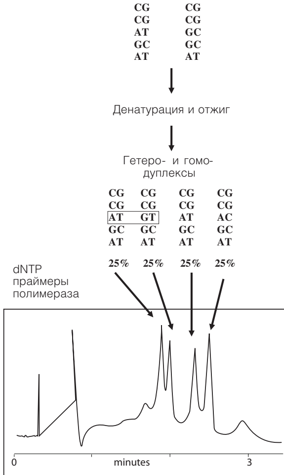
Рис. 4.6. Схема проведения DHPLC-анализа (пояснения в тексте)
