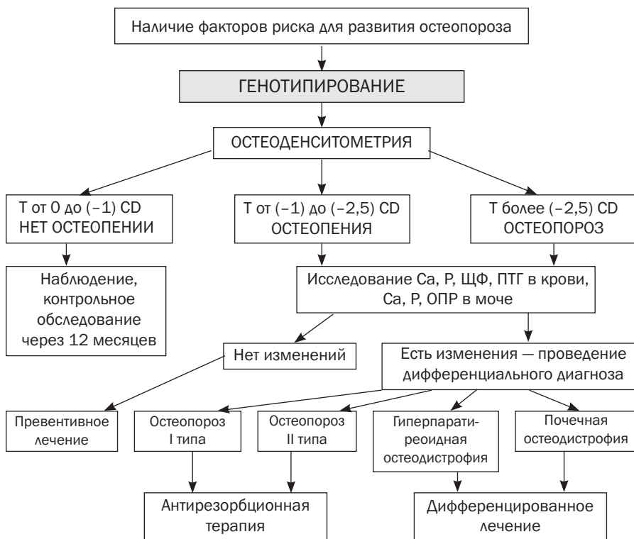
Рис. 6.2.7. Алгоритм обследования пациенток для диагностики остеопении
