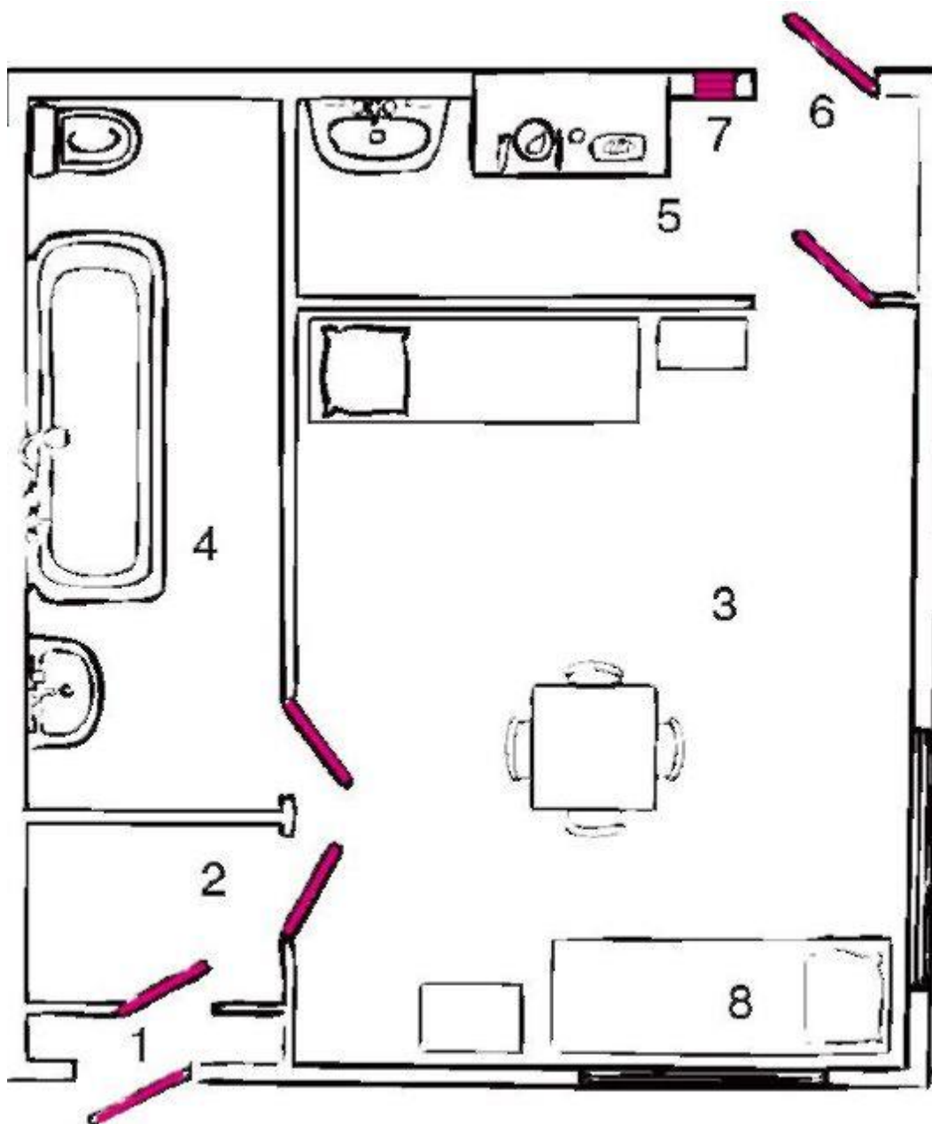
Рис. 3. План мельцеровского бокса:
